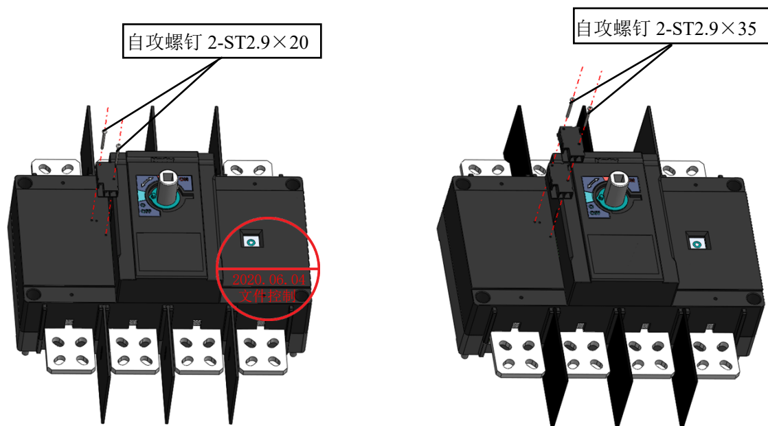
辅助触头安装（一个）
