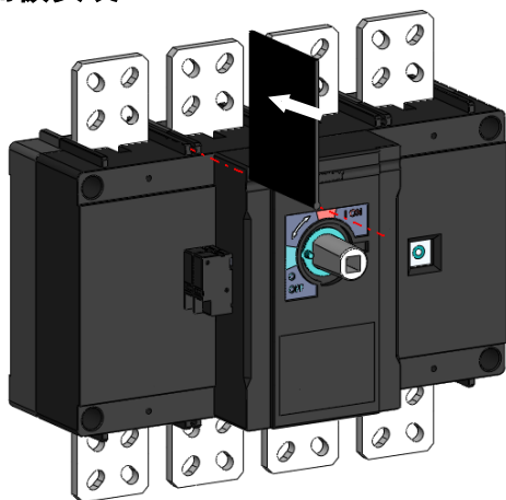
基本型产品相间隔板安装
